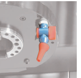
切屑吹气（喷嘴式）
