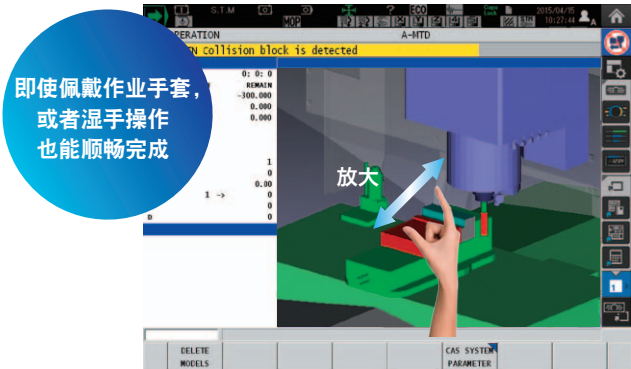
※上图所示Collision Avoidance System (特殊规格) 的画面示例
