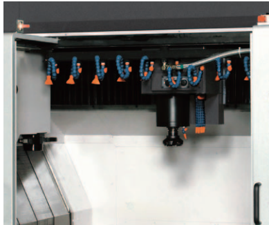
喷淋冲洗装置（安装顶盖规格）
