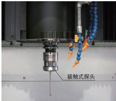
自动原点补偿、自动测量 （光电信号传达式接触式探头）
