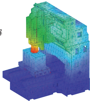
FEM有限元解析
